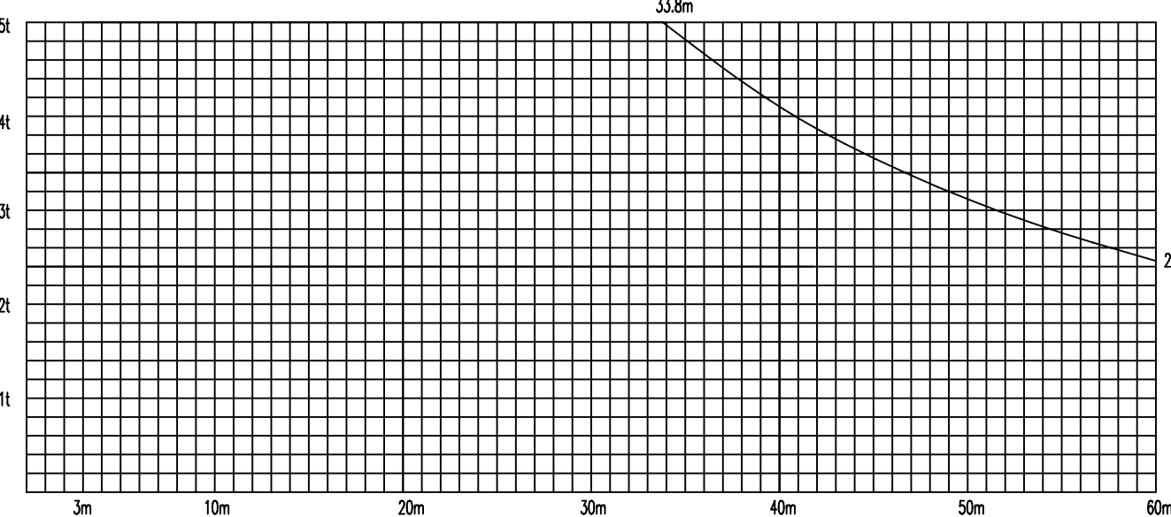
TC6024(QTZ160) 起升力矩曲线 (2倍率)
