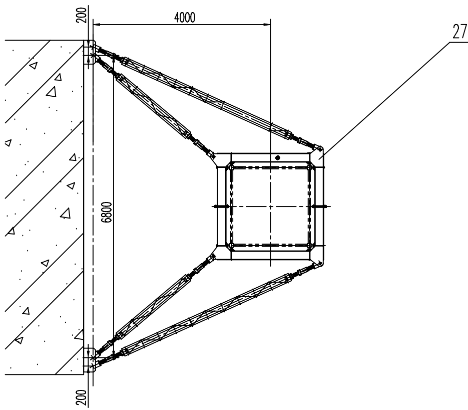
附墙架安装示意图
