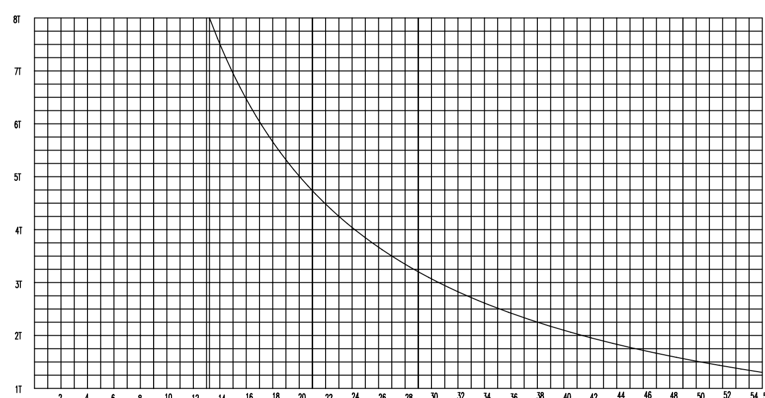
TC5513 起升力矩曲线(4倍率)
