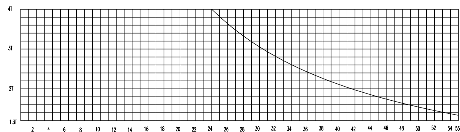
TC5513 起升力矩曲线(2倍率)
