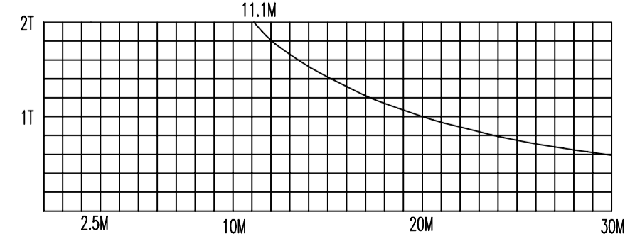
TC3006(QTZ20) 起升力矩曲线
